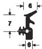
EPDM 4835
