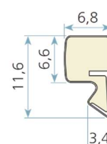
Q-lon 3005
